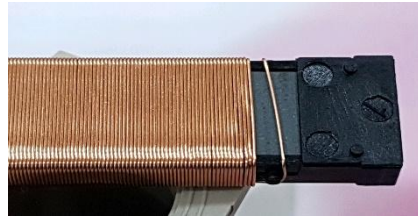
안테나코일 제품
