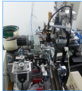
권선기
