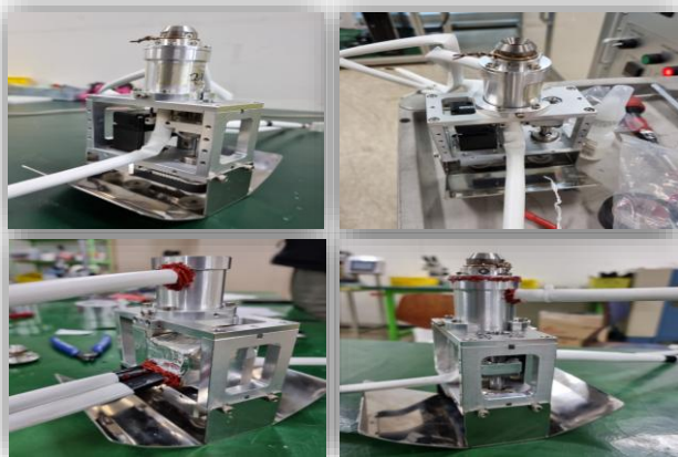
진공 챔버 내 추력기 동작 TESTER 기
